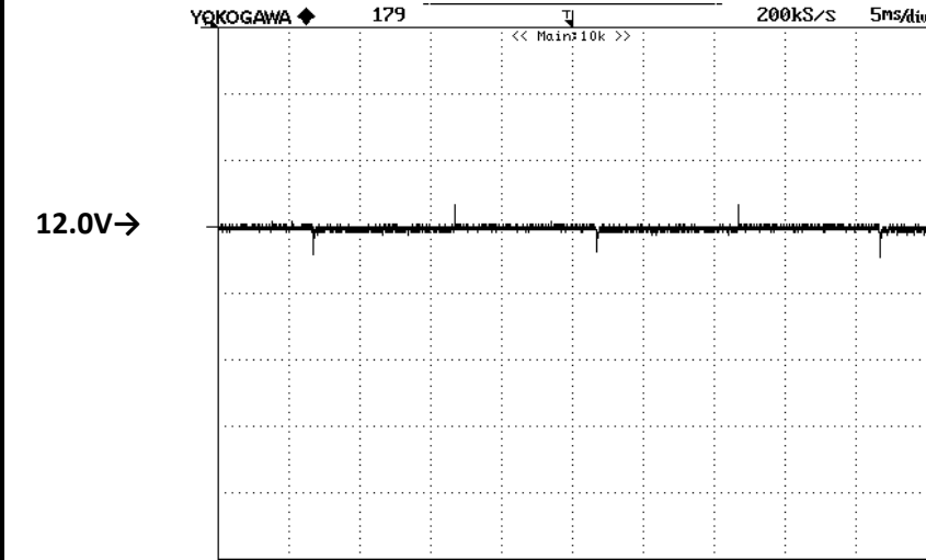
図12 タイミング時の負荷波形 Fig.12 Dynamic Load Waveform
