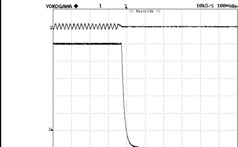
図14 出力電圧立下り波形 Fig.14 Output Voltage Falling Waveform
