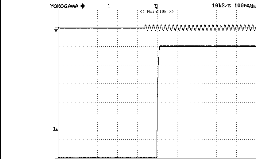
図13 出力電圧立上り波形 Fig.13 Output Voltage Rising Waveform
