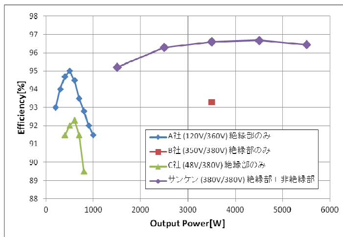
500V仕様 効率特性 (電源除く)
