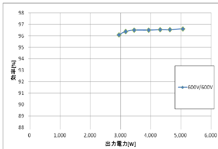
700V仕様 効率特性 (電源除く)
